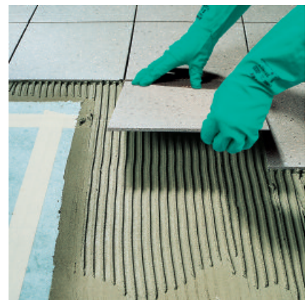
6. ... weitestgehend hohlraumfrei verlegen.
