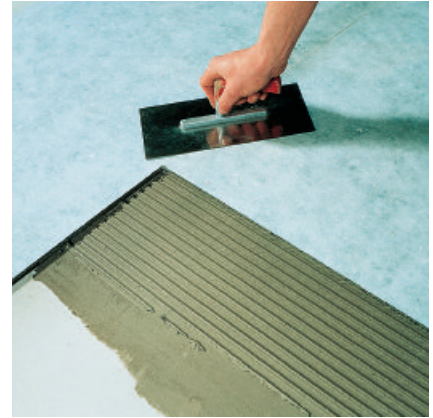
3. ... und mit einer Glättkelle andrücken.
