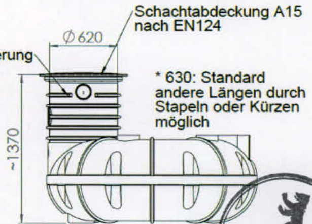
Begehbare Version mit Schacht- verlängerung und Schacht- abdeckung A15 aus Gusseisen (nicht geregeltes Zubehör)
