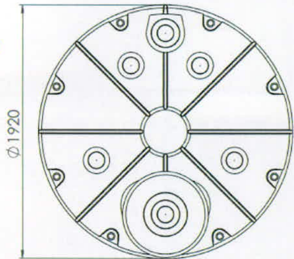
Draufsicht
