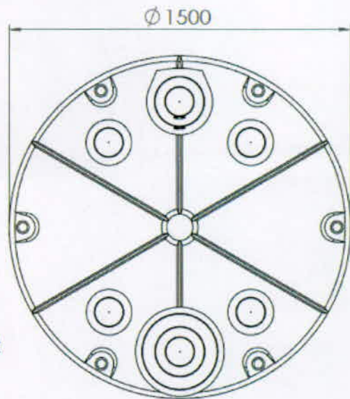
Draufsicht
