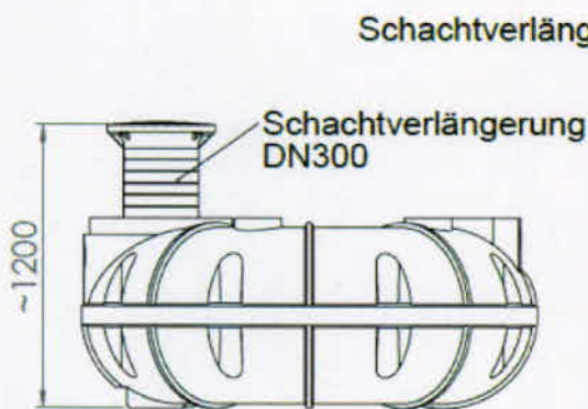
Begehbare Version mit Schacht- verlängerung und Schacht- abdeckung (nicht geregeltes Zubehör)
