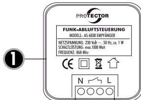
ANSCHLUSSBEISPIEL 1
