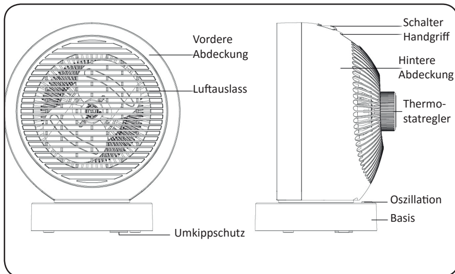
Abb. 2: Geräteübersicht (HHL 2000/3/3 O)
