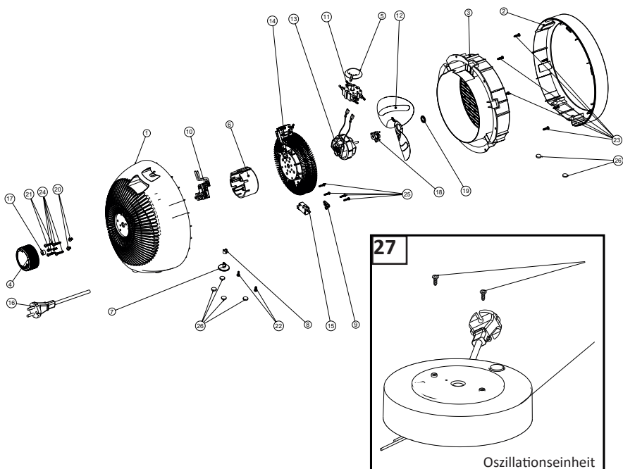
Abb. 3: Explosionszeichnung
