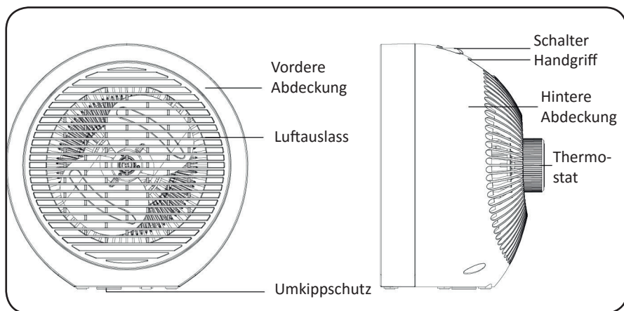
Abb. 1: Geräteübersicht (HHL 2000/3/3)
